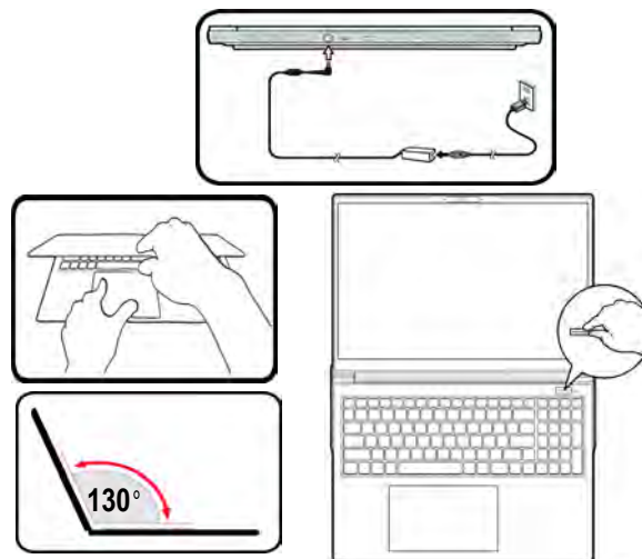
Abb. 1 - Öffnen des Deckels/Computers mit angeschlossenem AC/DC-Adapter
