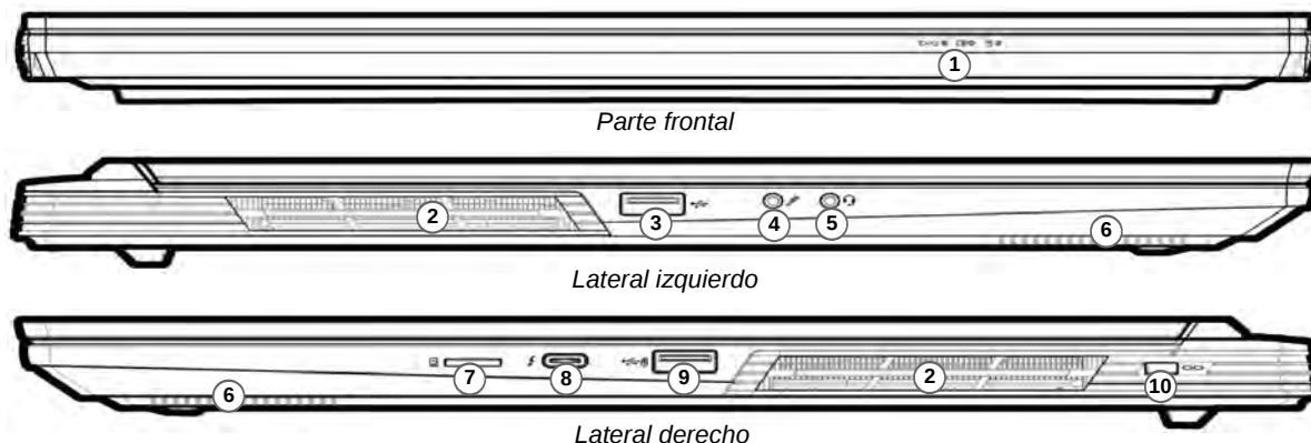
Figura 3 - Vistas frontal, izquierda y derecha
