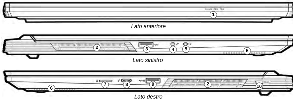
Figura 3 - Vista anteriore, sinistra e destra
