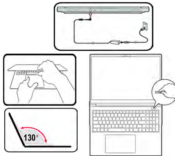
Figura 1 - Apertura del coperchio/Computer con alimentatore AC/DC collegato
