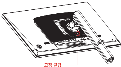
고정 클립
